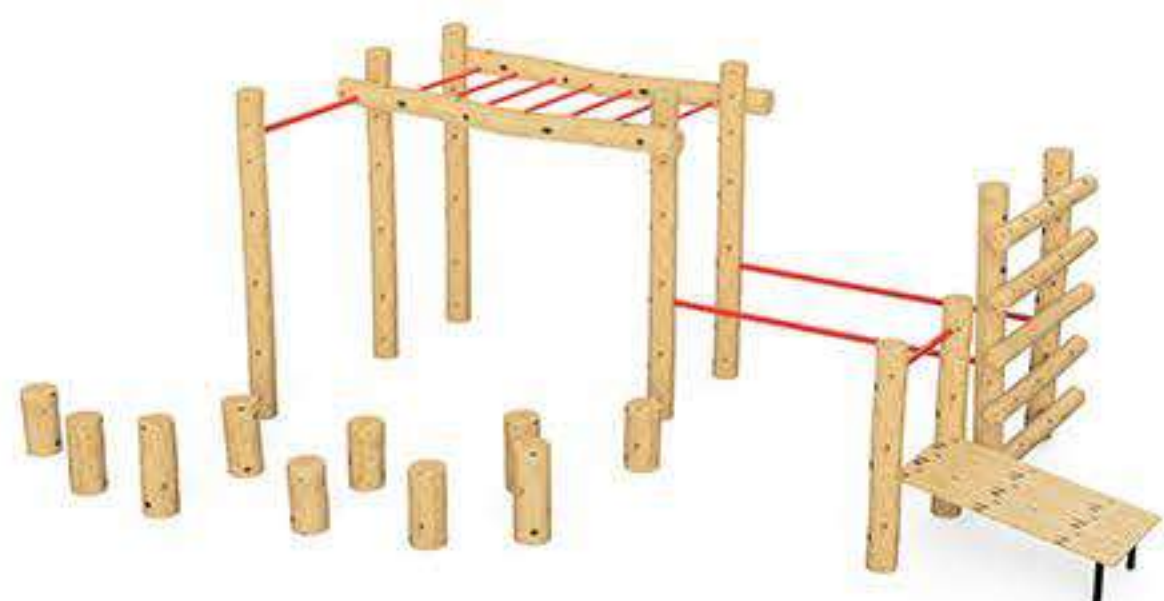
PTA - 06 Tor Przeszkód Marzenie Strefa bezpieczeństwa: 13,1 x 12,33 m
