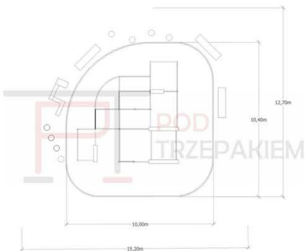
RYSUNEK TECHNICZNY:
